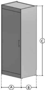
1 door armoire
